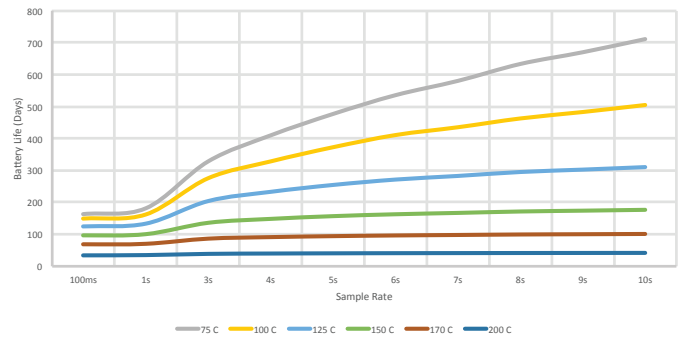
Gen 2 Quartz: VHT 200 4C
