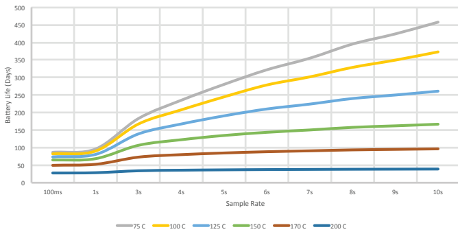
Gen 2 Quartz: VHT 200 2C
